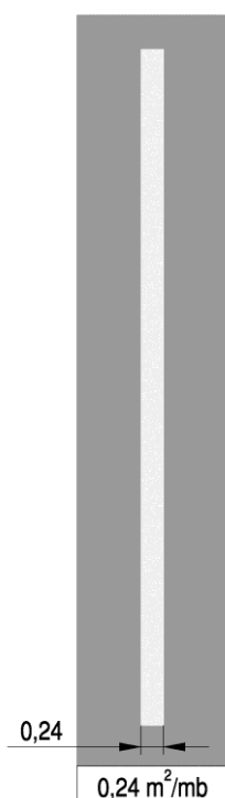
Rys. 2.2.2.4. Znak P-7b
