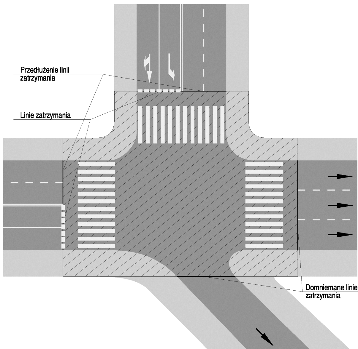
Rys. 2.1.1. Obszar skrzyżowania
