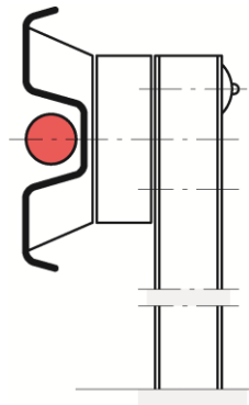
Rys. 2.1.4. Przykład punkтового elementu odbłaskowego U-1c umieszczanego na barierze ochronnej
