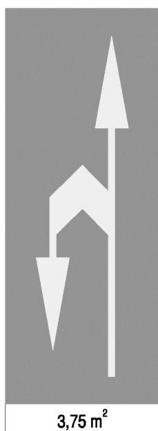
Rys. 3.2.1.10. Znak P-8i
