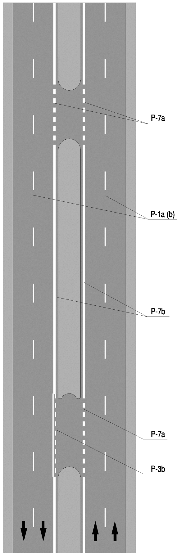
Rys. 7.2.9. Oznakowanie przejazdów przez pas dzielący jezdnie
