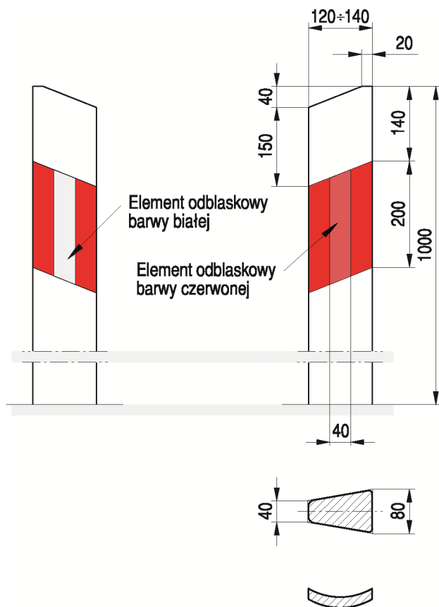
Rys. 2.1.1.1. Wzory słupków prowadzących U-1a umieszczanych samodzielnie na poboczu
