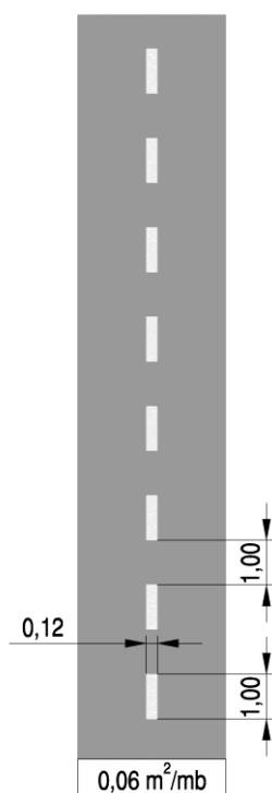
Rys. 2.2.2.3. Znak P-7c
