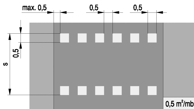
Rys. 4.2.2.1. Znak P-11:
