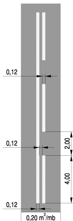
Rys. 2.2.1.8. Znak P-3a
