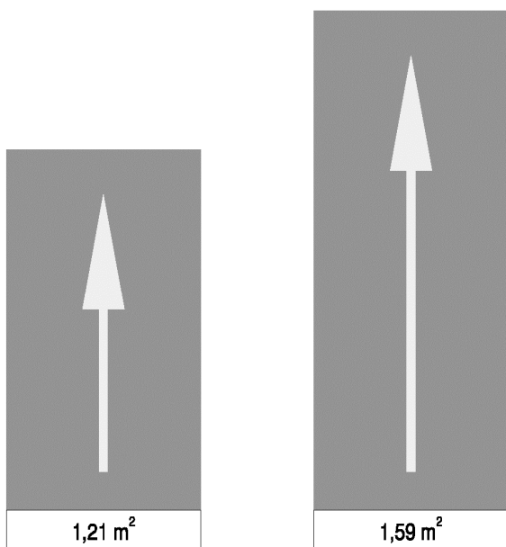
Rys. 3.2.1.2. Znak P-8a:
