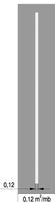
Rys. 2.2.2.5. Znak P-7d
