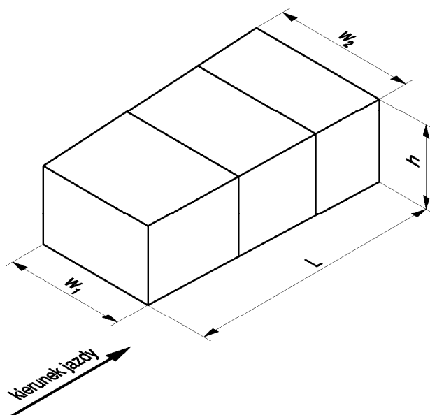
Rys. 7.2.1. Oslona energochłonna wielosegmentowa U-15a
