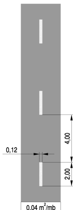
Rys. 2.2.1.2. Znak P-1b
