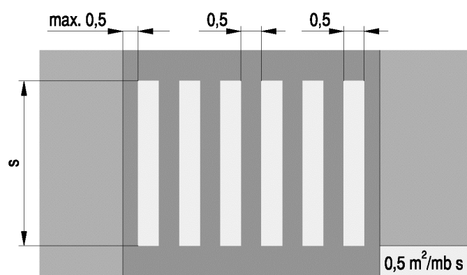
Rys. 4.2.1.1. Znak P-10:
