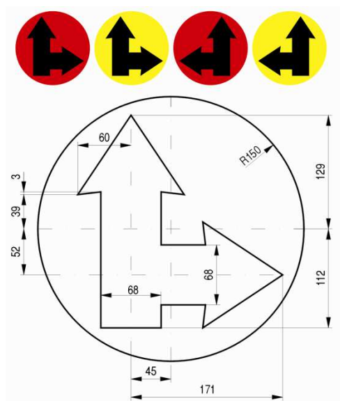
Rys. 10.5. Strzałki kierunku jazdy na wprost i w prawo lub na wprost i w lewo (odbicie zwierciadlane) dla sygnału czerwonego i żółtego. Symbol strzałek na wprost i w lewo obrócony o 90° w lewo dotyczy jazdy w lewo i zawracania
