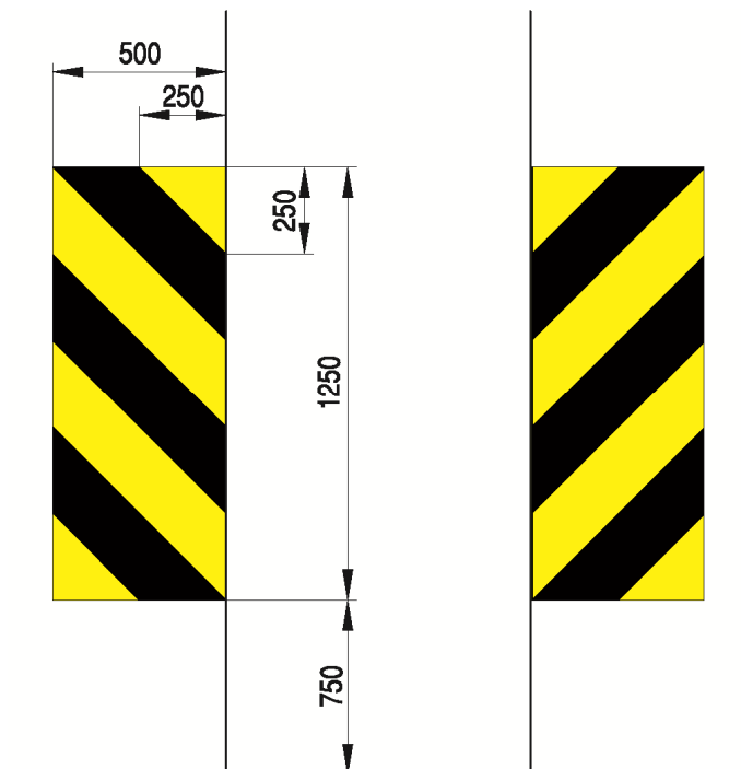
a) tablica U-9a
