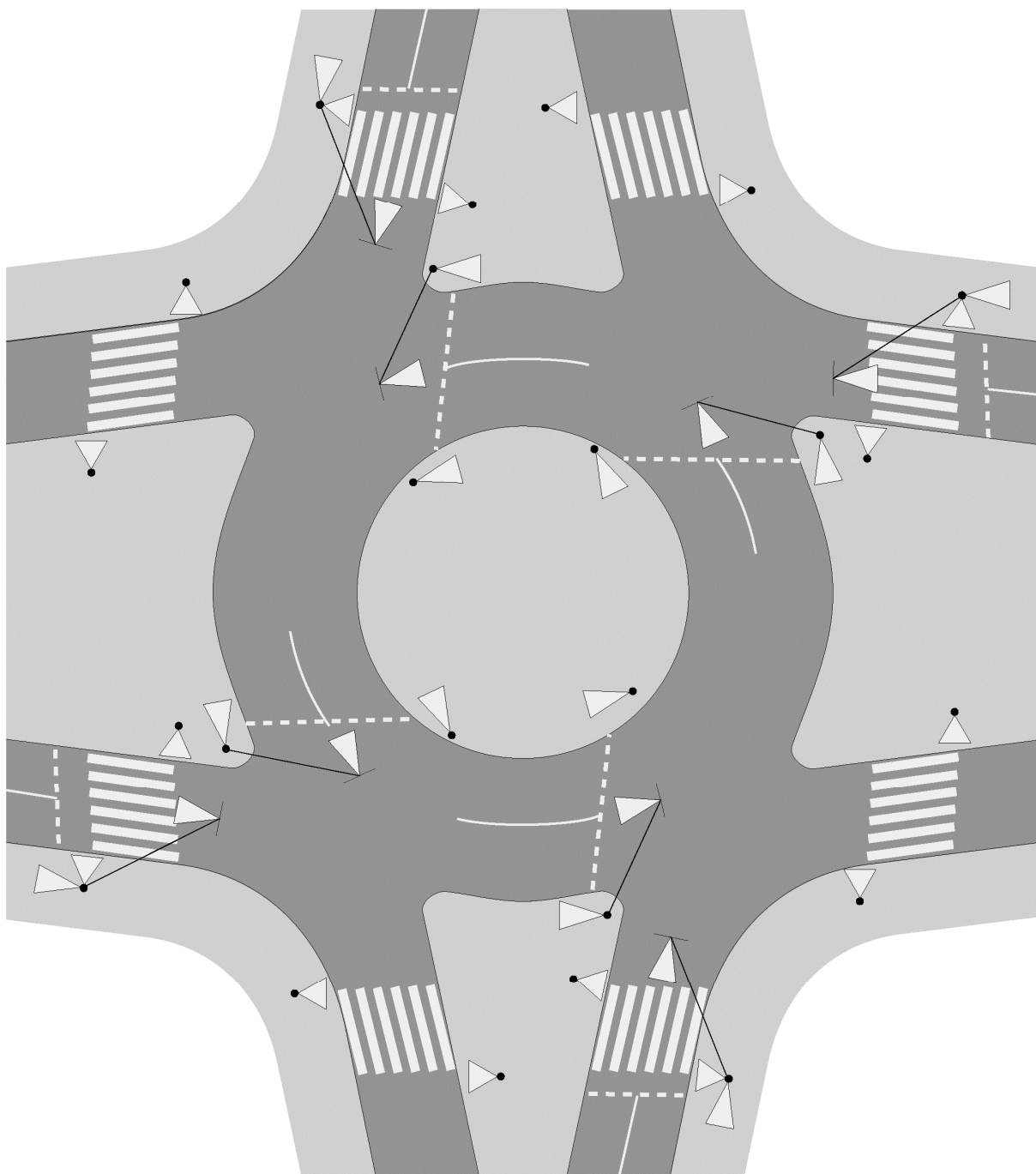
Rys. 7.3.8. Przykład lokalizacji sygnalizatorów na skrzyżowaniu z ruchem okrężnym o wlotach dwupasowych
