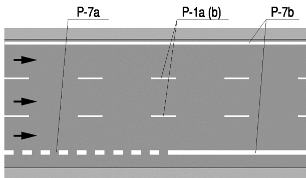
Rys. 7.2.5. Oznakowanie jezdni jednokierunkowej trzypasowej:
