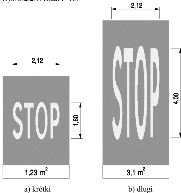
Rys. 5.2.2.1. Znak P-16:
